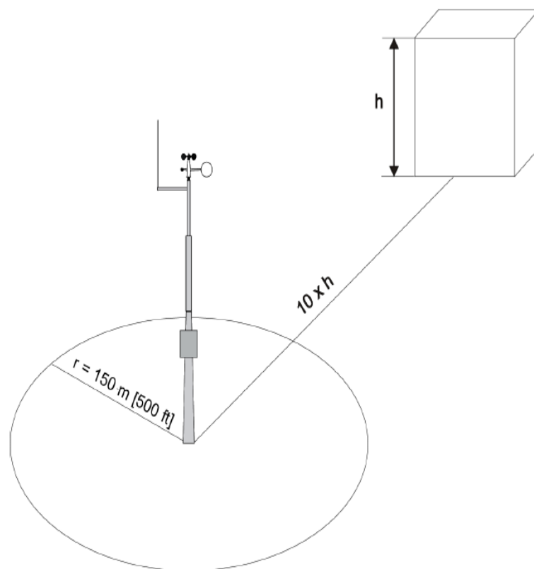
รูปที่ ๒๔ ขอบเขตพื้นที่ติดตั้งสถานี
