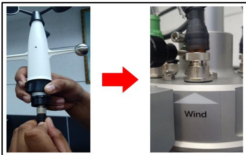
รูปที่ ๘๖ จุดเชื่อมต่อสัญญาณเครื่องวัดทิศทางและความเร็วลม
