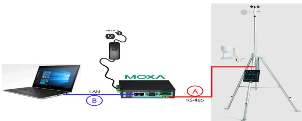
รูปที่ ๒๑ แสดงการเชื่อมต่อ (Simplified Connection)
