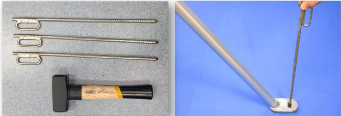
รูปที่ ๑๖ ชุดสมอบก (Ground peg)
