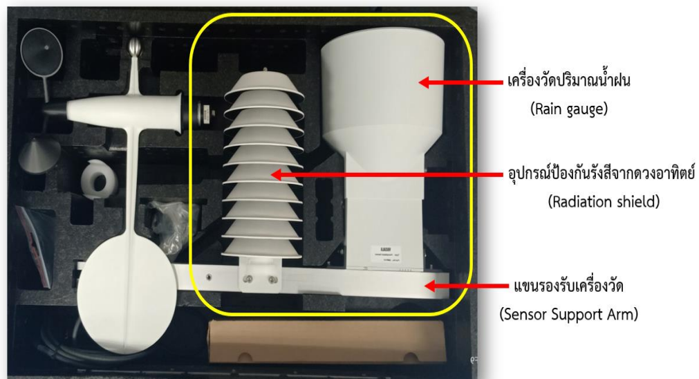
รูปที่ ๓๒ ชุดแขนรองรับเครื่องวัดที่เก็บอยู่ในกระเป๋า
