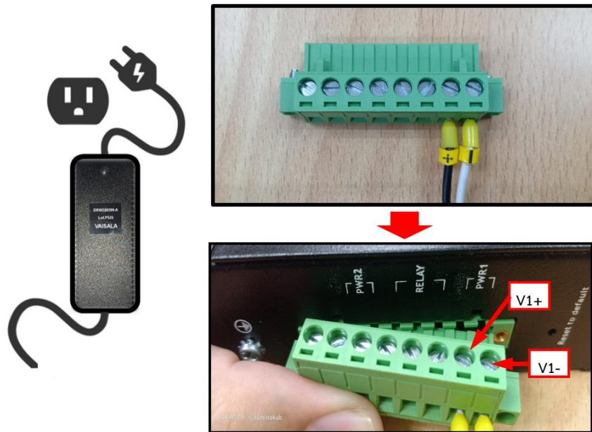
รูปที่ ๕๐ เชื่อมต่อแหล่งจ่ายไฟให้อุปกรณ์แปลงสัญญาณ (MOXA)
