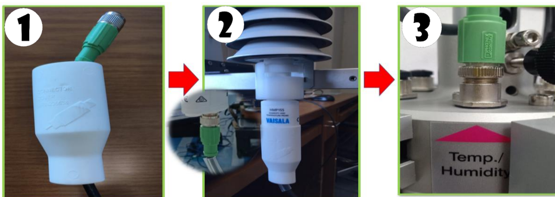
รูปที่ ๓๙ การต่อสายสัญญาณสำหรับเครื่องวัดอุณหภูมิและความชื้นสัมพัทธ์
