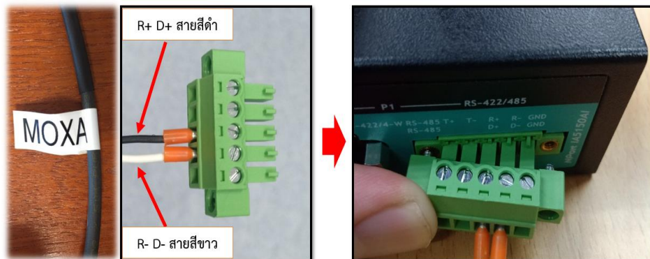
รูปที่ ๔๙ เชื่อมต่อสายสัญญาณกับอุปกรณ์แปลงสัญญาณ
