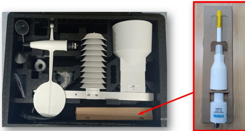
รูปที่ ๓๔ ชุดเครื่องวัดอุณหภูมิและความชื้นสัมพัทธ์
