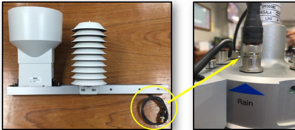
รูปที่ ๔๐ การเชื่อมต่อเครื่องวัดปริมาณน้ำฝน
