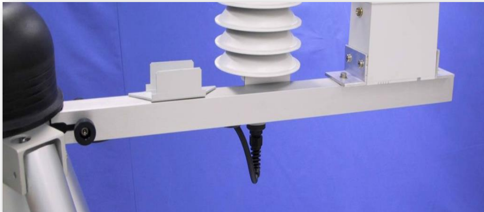
รูปที่ ๔ แขนรองรับเครื่องวัด (QMA101)
